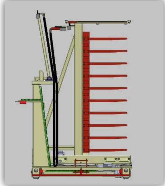
(25) – FORKLİFT 3 TON – DİESEL / ÜRETİM İÇİN h: 4,20 mt.
